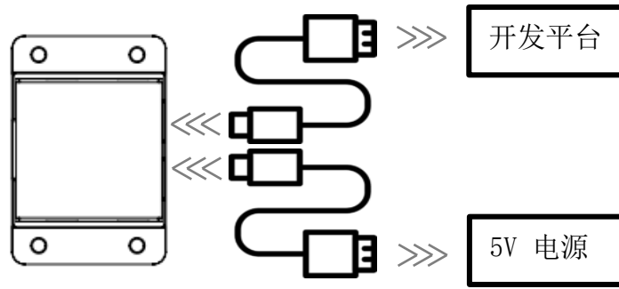
图 4 YDLIDAR G4 辅助供电
