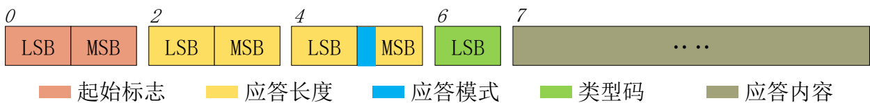
图 3 YDLIDAR TEA 雷达系统报文数据协议示意图
