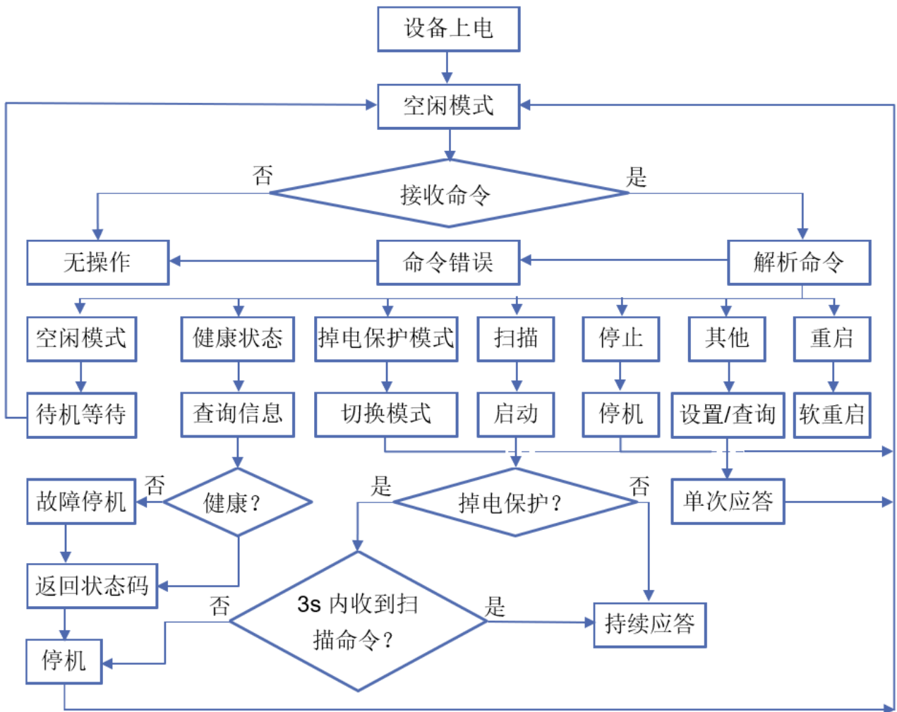
图 1 YDLIDAR TEA 雷达系统工作流程图
