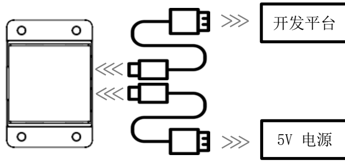
图 4 YDLIDAR G1 辅助供电
