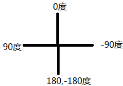
图 24 YDLIDAR G2 坐标角度定义
