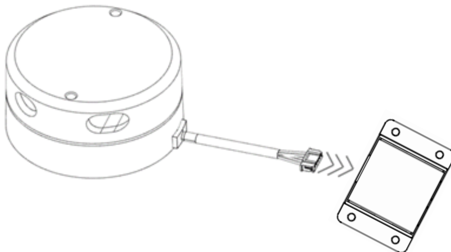
图 2 YDLIDAR G2 设备连接 STEP 1
