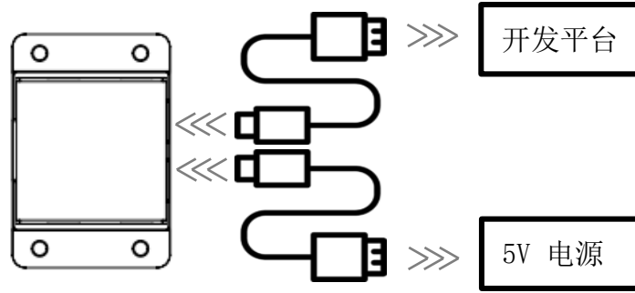
图 4 YDLIDAR G2 辅助供电
