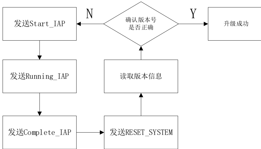
图 8 升级流程图
