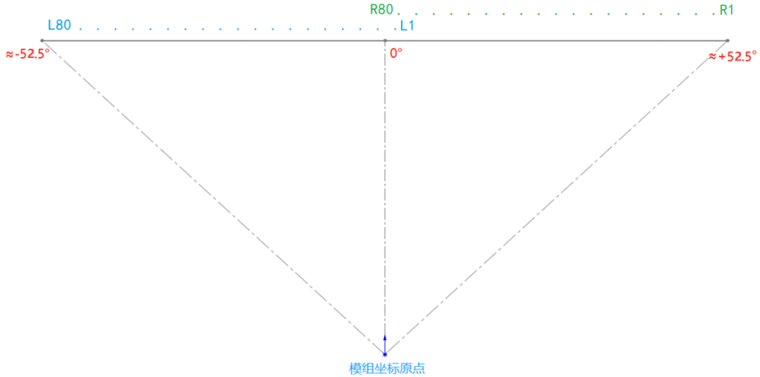
图 2 YDLIDAR GS2 输出点云角度示意图
