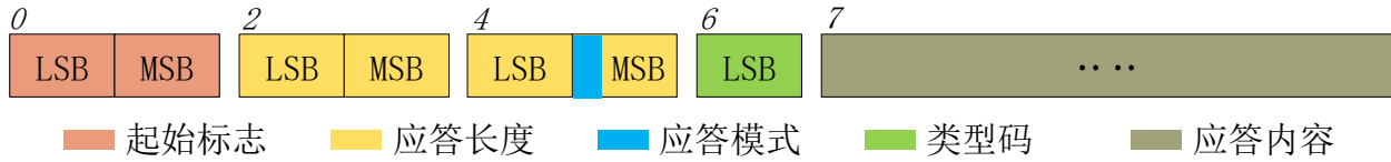
图 3 YDLIDAR X4 系统报文数据协议示意图
