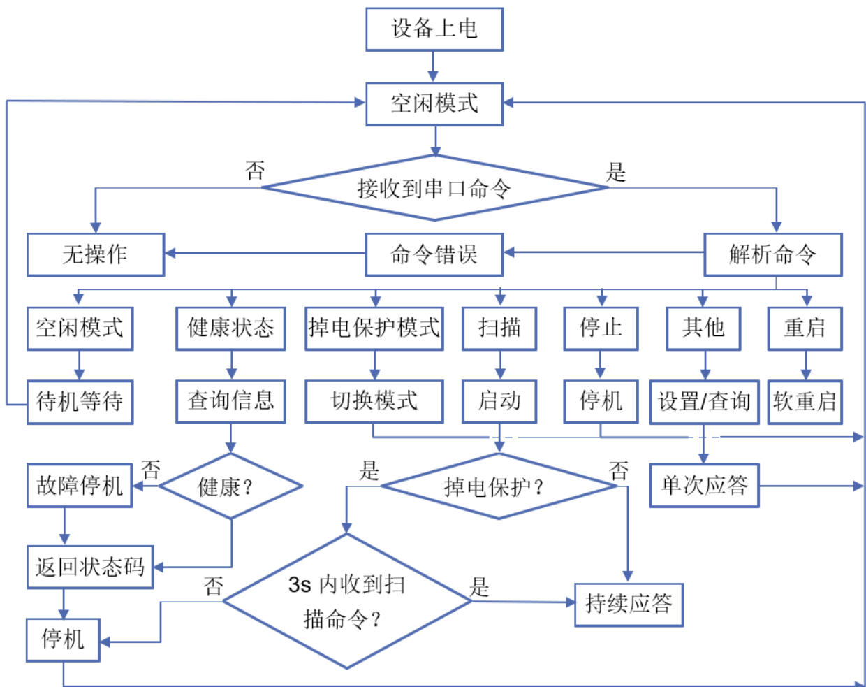
图 1 YDLIDAR G4 系统工作流程图
