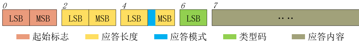
图 3 YDLIDAR G4 系统报文数据协议示意图
