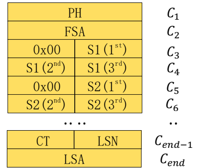
图 8 CS 异或顺序示意图
