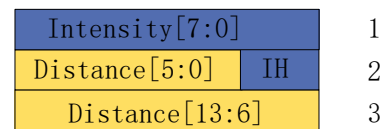
图 6 S 节点数据结构示意图
