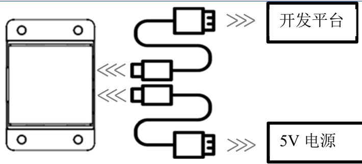
图 4 YDLIDAR G6 辅助供电
